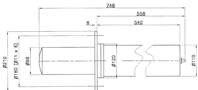
Type ORT-S4-F500
