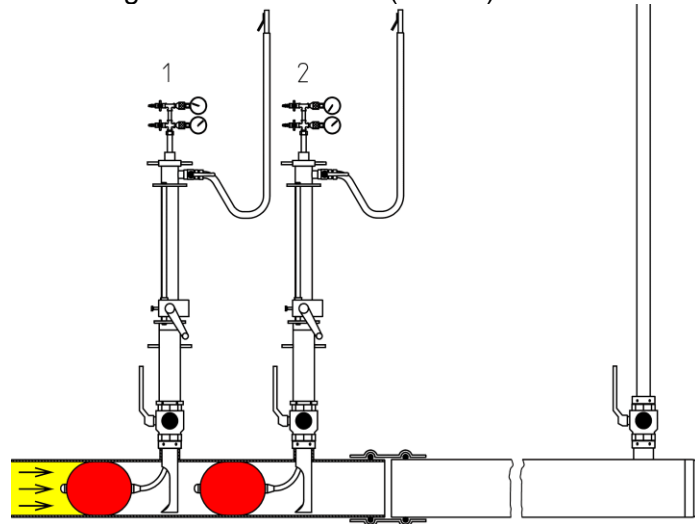
Afb. 1 Situatie afsluiting
