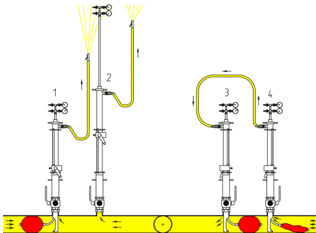
Druknivellering met by-pass 2" bij lange afstanden
