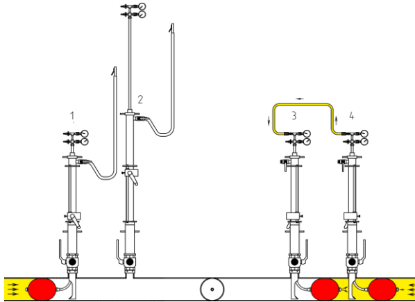
Afb. 2 Blaas (apparaat 2) trekken, omdat beide zijden drukloos zijn. Door de voordrukmeting van apparaat 3 en 4 de druk nivelleren aan beide zijden van de blaas van apparaat 4.
