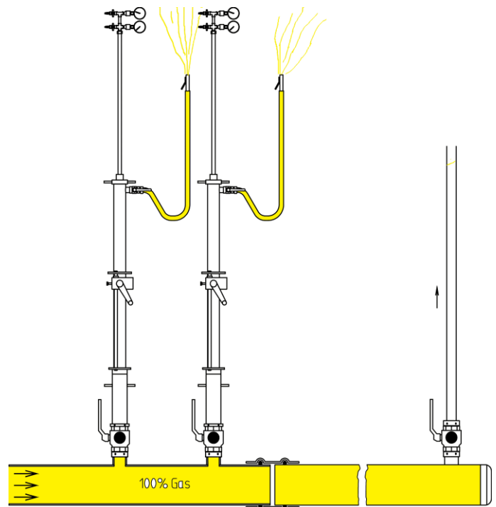
Afb. 3 De druk van de 1e blaas aflaten en beide blazen in de lans terugtrekken. Het apparaat uit de leiding halen. Leiding ontluichten tot er 100% gas gemeten wordt.
