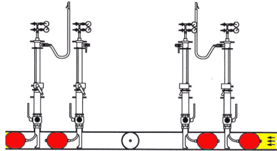
Afb. 2 Blaas (apparaat 2) trekken, omdat beide zijden drukloos zijn. Door de voordrukmeting van apparaat 3 en 4 de druk nivelleren aan beide zijden van de blaas van apparaat 4.
