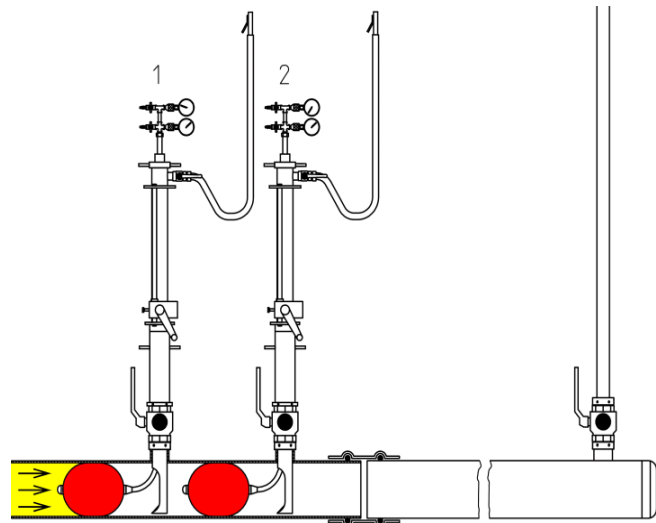
Afb.1 Situatie afsluiting
