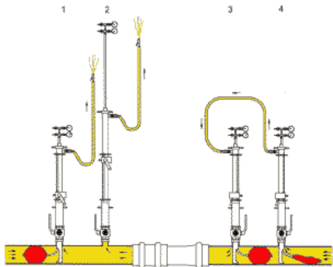
Afb. 3 De druk van de blaas (apparaat 4) afdrukken. Druknivellering van de werkplek d.m.v. een overbruggings slang van apparaat 4 naar 3. De werkplek ontluichten via de ontluichtings slang van apparaat 1 en 2. Nadat de ontluichtingskranen van apparaat 1 en 2 weer gesloten zijn kunnen de resterende blazen getrokken worden.
