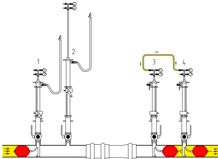
Afb. 2 De druk van blaas afdrukken (apparaat 2), omdat beide zijden drukloos zijn. Door de voordrukmeting van apparaat 3 en 4 de druk nivelleren aan beide zijden van de blaas van apparaat 4.
