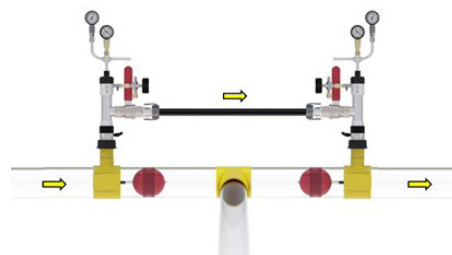
Het creëren van een by-pass.
