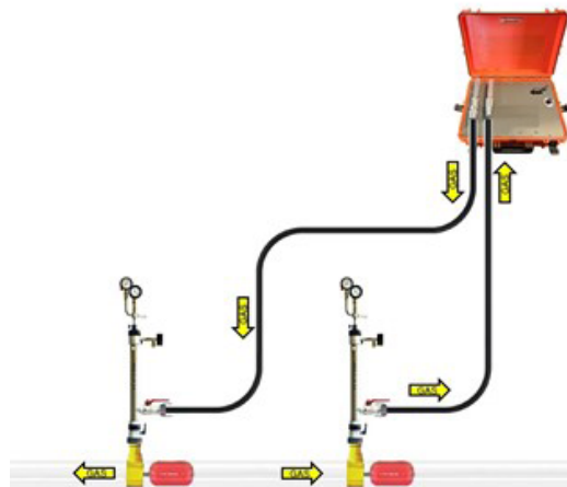
Gas uit leidingsecties overpompen naar het net.
