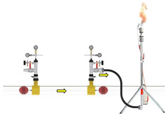
Spoelen/purgen van het leidingdeel tussen de blazen.
