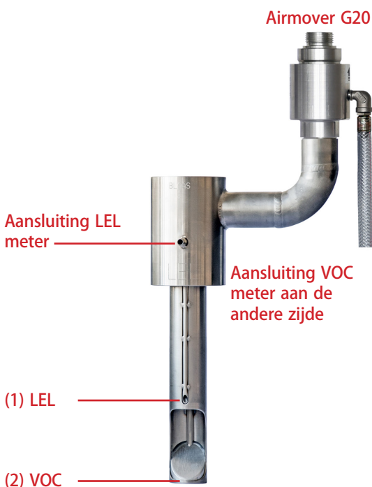
De afgebeelde zakbuis is t.b.v. een 4" leiding i.c.m. een 2" TOR nipple.
